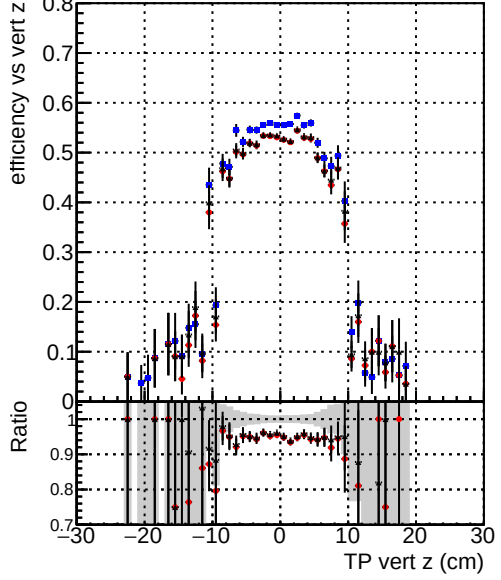
Efficiency vs vert z — DQMstep3_TT_CKF — DQMstep3_TT_default — DQMstep3_TT_defaultNEWTepo7
