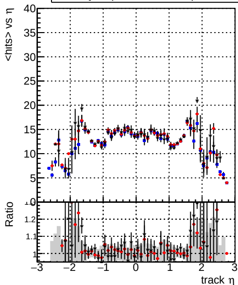
mean hit DQMstep3_TT_CKF DQMstep3_TT_default DQMstep3_TT_defaultNEWTepo7
