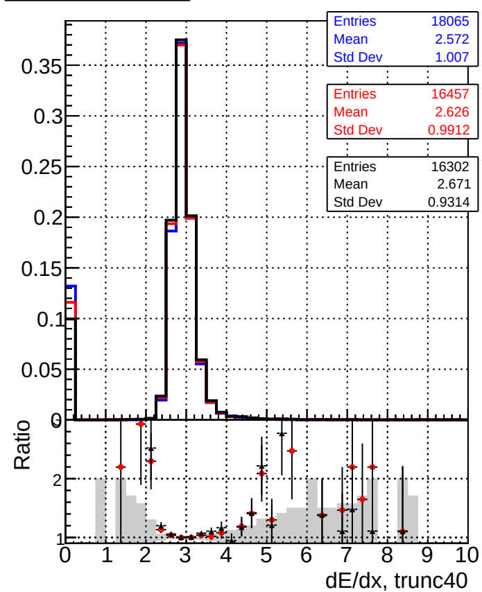
— DQMstep3 TT CKF — DQMstep3 TT default — DQMstep3 TT defaultNEWTepo7
