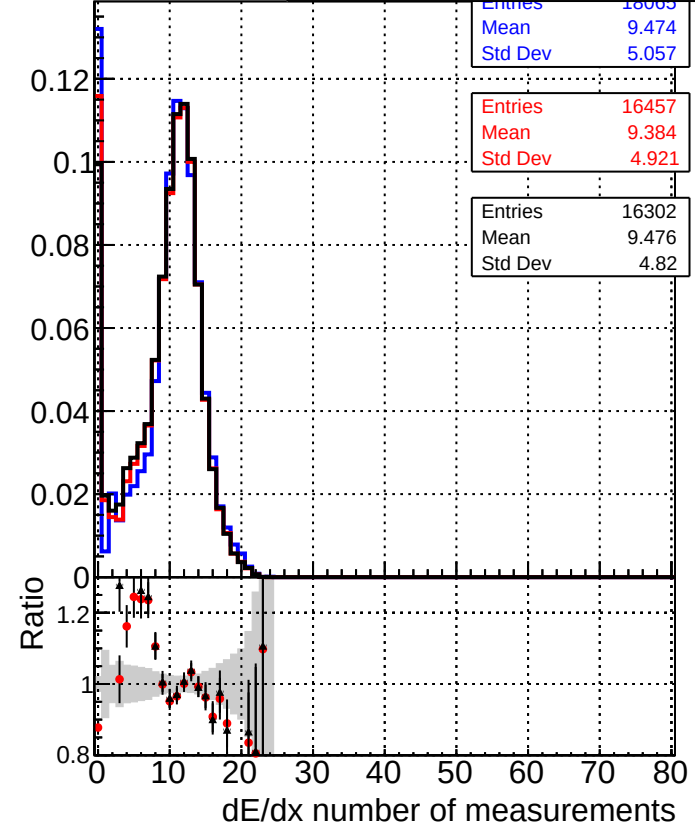
— DQMstep3 TT CKF — DQMstep3 TT default — DQMstep3 TT defaultNEWTepo7
