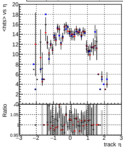
mean hits vs \eta Legend: DQMstep3_TT_CKF (blue), DQMstep3_TT_default (red), DQMstep3_TT_defaultNEWTepo7 (black)
