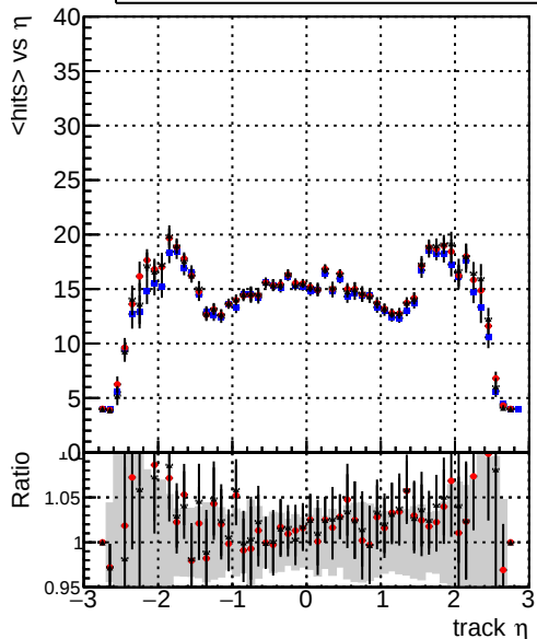
— DQMstep3_TT_CKF — DQMstep3_TT_default — DQMstep3_TT_defaultNEWTepo7 mean hit
