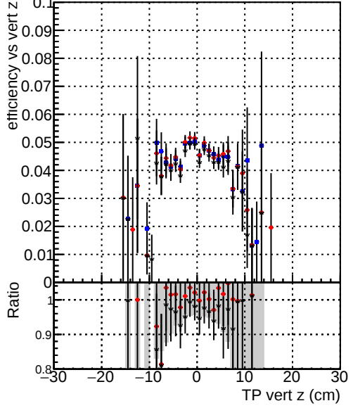
Efficiency vs. TP vert z (cm) Legend: - DQMstep3_TT_CKF (blue circles) - DQMstep3_TT_default (red circles) - DQMstep3_TT_defaultNEWTepo7 (grey circles)
