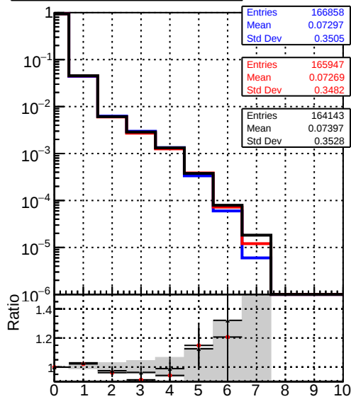
mean hits — DQMstep3_TT_CKF — DQMstep3_TT_default — DQMstep3_TT_defaultNEWTepo7
