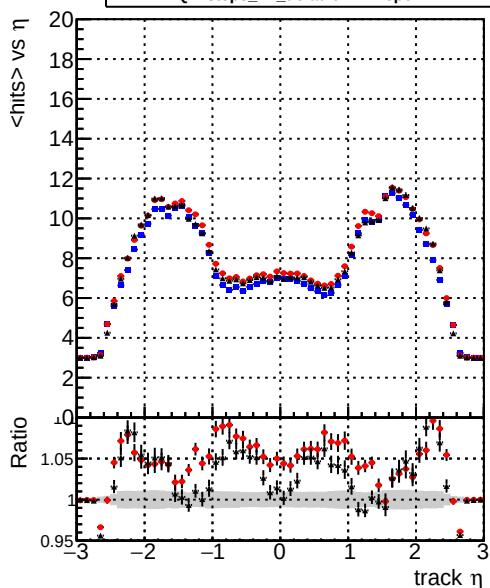
mean hits — DQMstep3_TT_CKF — DQMstep3_TT_default — DQMstep3_TT_defaultNEWTepo7
