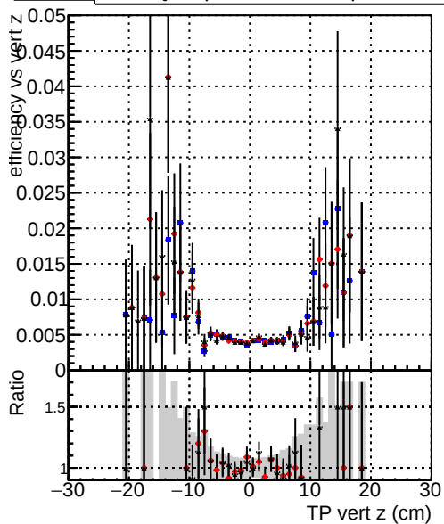
Efficiency vs. sim PV z — DQMstep3_TT_CKF — DQMstep3_TT_default — DQMstep3_TT_defaultNEWTepo7
