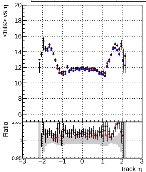
DQMstep3_TT_CKF DQMstep3_TT_default DQMstep3_TT_defaultNEWTepo7 mean hit
