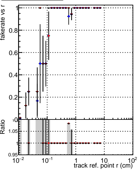
—•— DQMstep3_TT_CKF —•— DQMstep3_TT_default —•— DQMstep3_TT_defaultNEWTEp07
