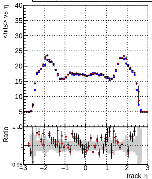
mean hits vs \eta — DQMstep3_TT_CKF — DQMstep3_TT_default — DQMstep3_TT_defaultNEWTepo7
