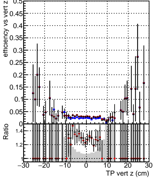
Efficiency vs vert z Legend: - DQMstep3_TT_CKF (blue stars) - DQMstep3_TT_default (red circles) - DQMstep3_TT_defaultNEWTepo10 (black crosses)
