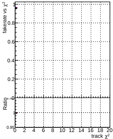
Fake rate vs. —●— DOMstep3 TT CKF —●— DOMstep3 default —●— DOMstep3 defaultNEWTepo10
