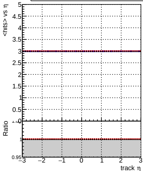
mean hits vs \eta DQMstep3_TT_CKF DQMstep3_TT_default DQMstep3_TT_defaultNEWTepo10
