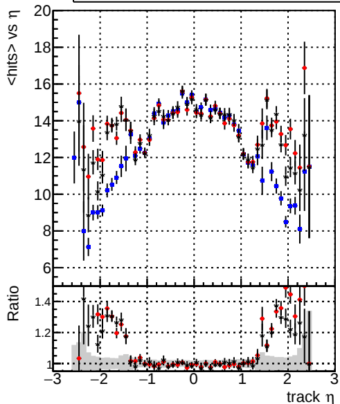
mean hit — DQMstep3_TT_CKF — DQMstep3_TT_default — DQMstep3_TT_defaultNEWTepo10
