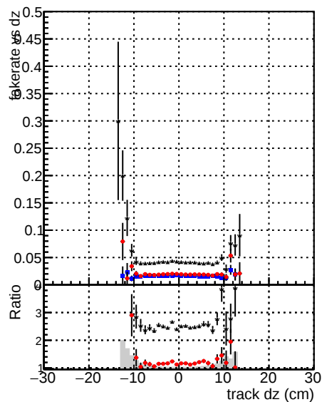
Fake rate vs d DOMstep3 TT CKF DOMstep3 TT default DOMstep3 TT defaultNEWTepo10
