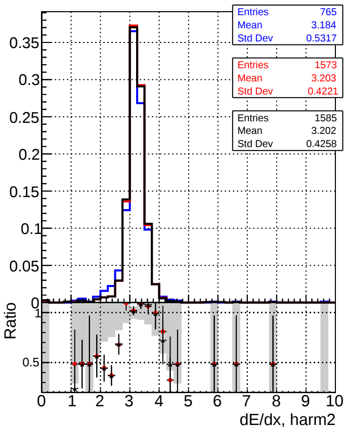
DQMstep3_TT_CKF DQMstep3_TT_default DQMstep3_TT_defaultNEWTep10
