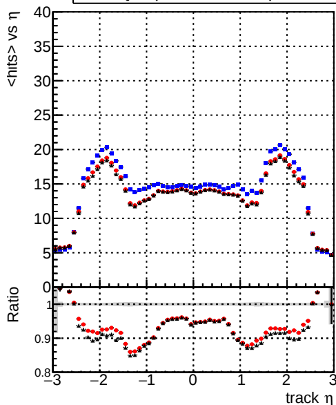
mean hits vs \eta — DQMstep3_TT_CKF — DQMstep3_TT_default — DQMstep3_TT_defaultNEWTepo10
