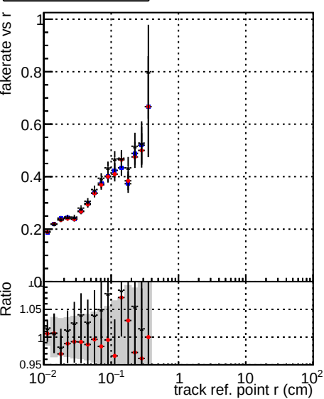
Fake rate vs verpos DOMstep3 TT CKF DOMstep3 TT default DOMstep3 TT defaultNEWTEpo10
