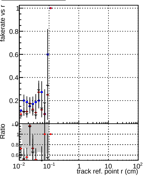
DOMstep3 TT CKF DOMstep3 TT default DOMstep3 TT defaultNEWTepo10
