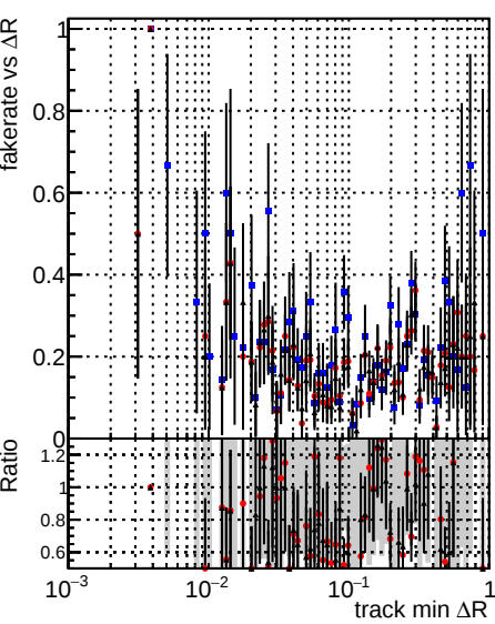
Legend: DQMstep3 TT CKF (blue dots), DQMstep3 TT default (red dots), DQMstep3 TT defaultNEWTepo10 (black line)
