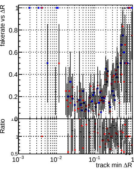
Legend: —●— DQMstep3_TT_CKF —●— DQMstep3_TT_default —●— DQMstep3_TT_defaultNEWTepo10
