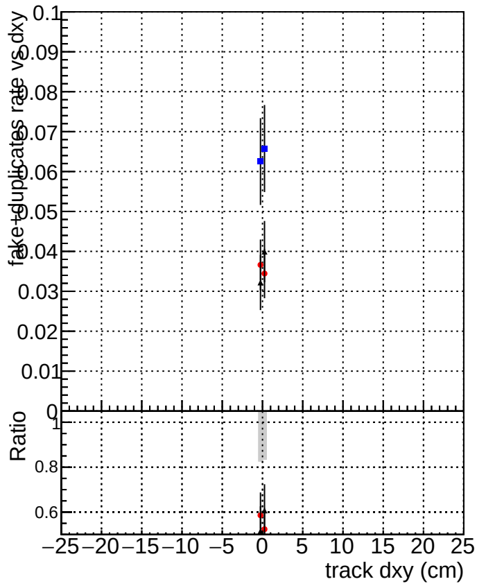
Legend for the plots: DQMstep3_TT_CKF (Blue squares) DQMstep3_TT_default (Red circles) DQMstep3_TT_defaultNEWTepo10 (Black stars)
