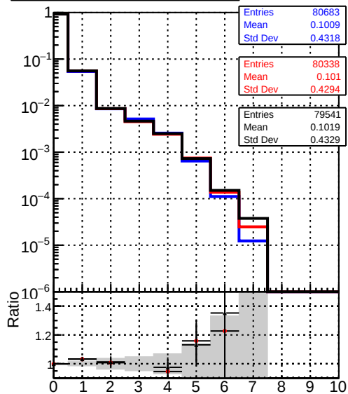
mean hit — DQMstep3_TT_CKF — DQMstep3_TT_default — DQMstep3_TT_defaultNEWTepo10
