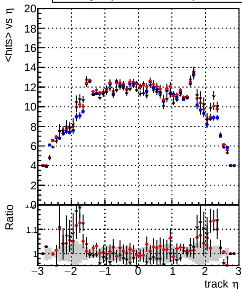
mean hits vs \eta Legend: DQMstep3_TT_CKF (blue), DQMstep3_TT_default (red), DQMstep3_TT_defaultNEWTepo10 (black)
