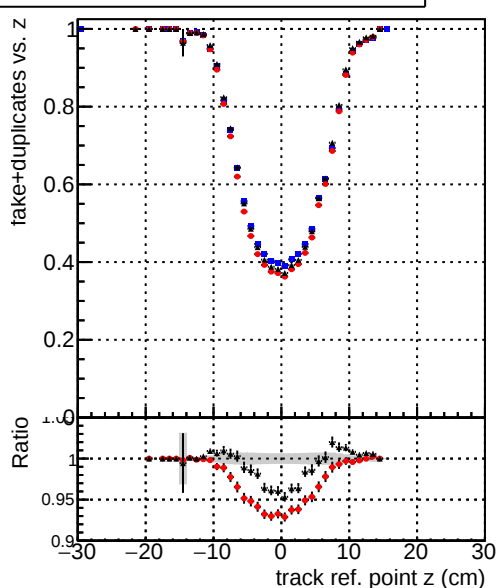
—●— DQMstep3_TT_CKF —●— DQMstep3_TT_default —●— DQMstep3_TT_defaultNEWTepo10
