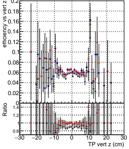
Efficiency vs. TP vert z Legend: - DQMstep3_TT_CKF (blue circles) - DQMstep3_TT_default (red circles) - DQMstep3_TT_defaultNEWTepo10 (black crosses)
