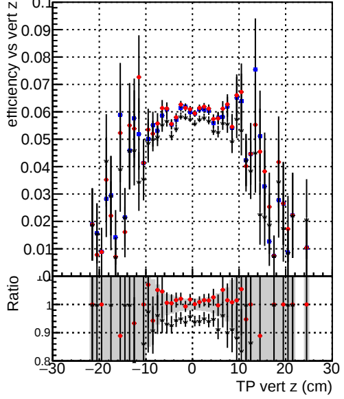
Efficiency vs. TP vert z (cm) —●— DQMstep3_TT_CKF —●— DQMstep3_TT_default —●— DQMstep3_TT_defaultNEWTepo10
