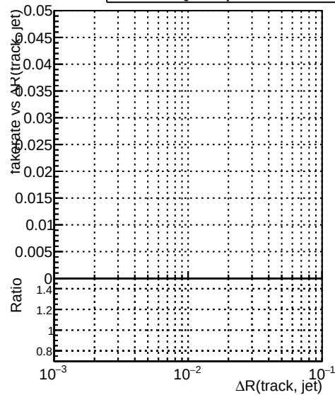
Legend: \blacksquare DQMstep3 TT CKF \bullet DQMstep3 TT default \times DQMstep3 TT defaultNEWTepo10
