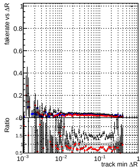
Legend: \blacksquare DQMstep3 TT CKF \bullet DQMstep3 TT default \times DQMstep3 TT defaultNEWTepo10
