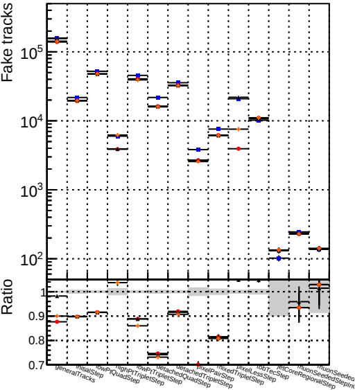
Number ■ DQMstep3 TT_CKF ● DQMstep3 TT_default ▲ DQMstep3 TT_ckfPixelLess ◆ DQMstep3 TT_default1
