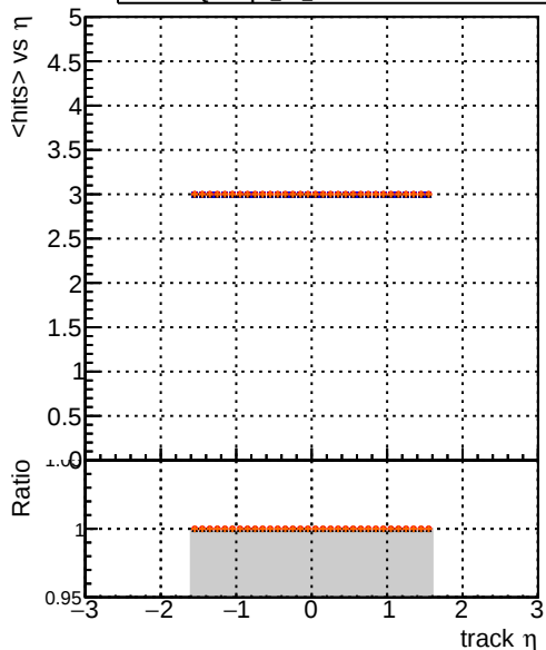
mean hit DQMstep3_TT_Ckf- DQMstep3_TT_default DQMstep3_TT_ckfPixelLess DQMstep3_TT_default1
