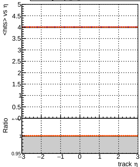
mean hits DQMstep3 TT CKF DQMstep3 TT default DQMstep3 TT ckfPixelLess DQMstep3 TT default1
