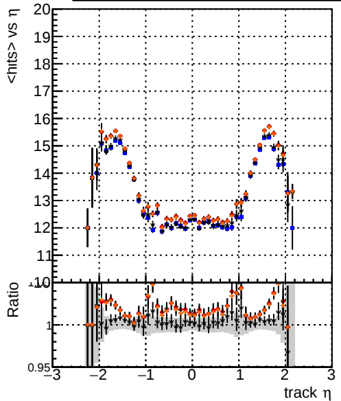
DQMstep3 TT CKF DQMstep3 TT default DQMstep3 TT_ckPixelLess DQMstep3 TT default1 mean hit
