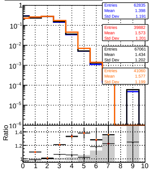
Legend: DQMstep3 TT CKF (blue), DQMstep3 TT_default (red), DQMstep3 TT_ckfPixelLess (black), DQMstep3 TT_default1 (orange) mean hit
