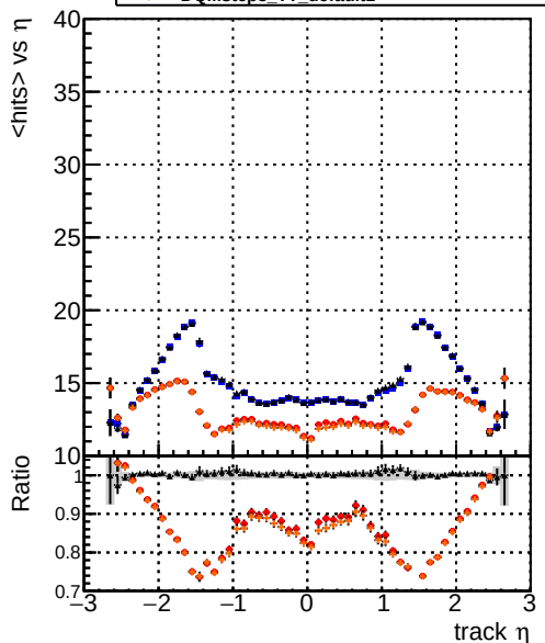
Legend: DQMstep3 TT CKF (blue), DQMstep3 TT_default (red), DQMstep3 TT_ckfPixelLess (black), DQMstep3 TT_default1 (orange) mean hit
