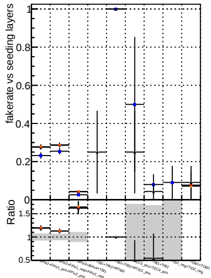
Fake rate vs. DOMstep3 DOMstep3+GKF DOMstep3+TEC4_pos default Less
