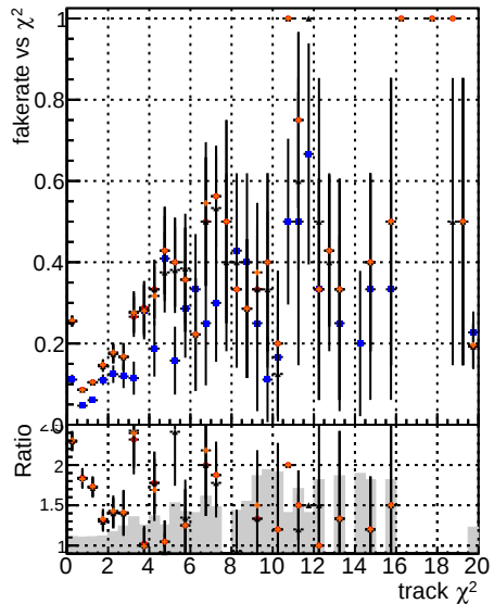
Fake rate vs. DOMstep3 DOMstep3+GKF DOMstep3+TEC4_pos default Less
