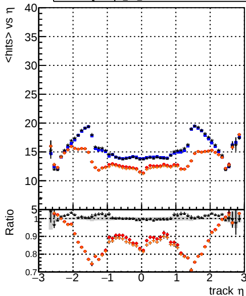
mean hits vs \eta DQMstep3 TT CKF DQMstep3 TT default DQMstep3 TT_ckfPixelLess DQMstep3 TT default1
