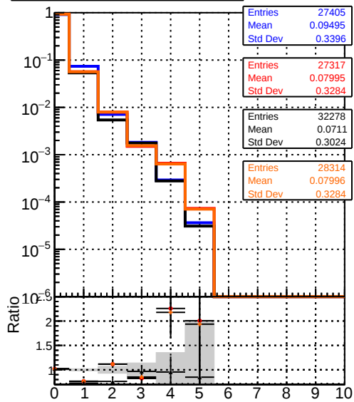
mean hits > \eta DQMstep3 TT CKF DQMstep3 TT default DQMstep3 TT ckfPixelLess DQMstep3 TT default1
