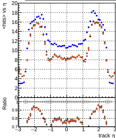
mean hits DQMstep3 TT CKF DQMstep3 TT default DQMstep3 TT_ckPixelLess DQMstep3 TT default1
