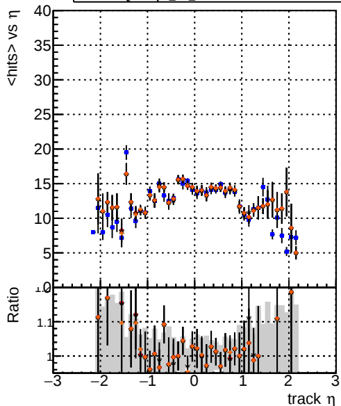
mean hits > \eta Legend: DQMstep3 TT CKF (blue), DQMstep3 TT default (red), DQMstep3 TT ckfPixelLess (black), DQMstep3 TT default1 (orange)
