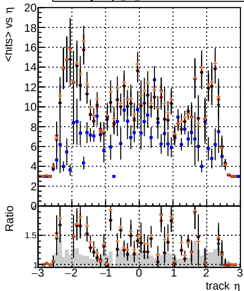
mean hits Legend: DQMstep3 TT CKF (blue), DQMstep3 TT default (red), DQMstep3 TT ckfPixelLess (black), DQMstep3 TT default1 (orange)
