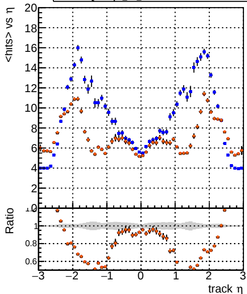
mean hits vs \eta Legend: Blue line: DQMstep3 TT CKF Red line: DQMstep3 TT default Black line: DQMstep3 TT_ckfPixelLess Orange line: DQMstep3 TT default1
