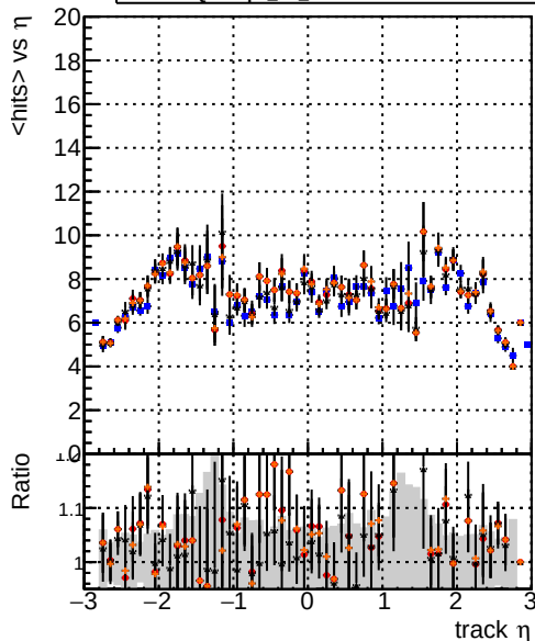
Legend: DOMstep3 TT CKF DOMstep3 TT default DOMstep3 TT_ckfPixelLess DOMstep3 TT default1 mean hits
