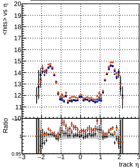
Legend: — DQMstep3 TT CKF — DQMstep3 TT_default — DQMstep3 TT_ckfPixelLess — DQMstep3 TT_default1
