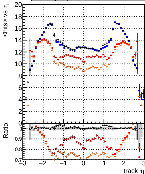
mean hits vs \eta Legend: DQMstep3 TT CKF (blue), DQMstep3 TT default (red), DQMstep3 TT ckfPixelLess (black), DQMstep3 TT default1 (orange)
