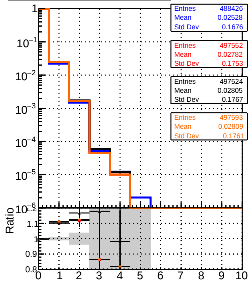
DQMstep3 TT CKF DQMstep3 TT_default DQMstep3 TT_ckfPixelLess DQMstep3 TT_default1
