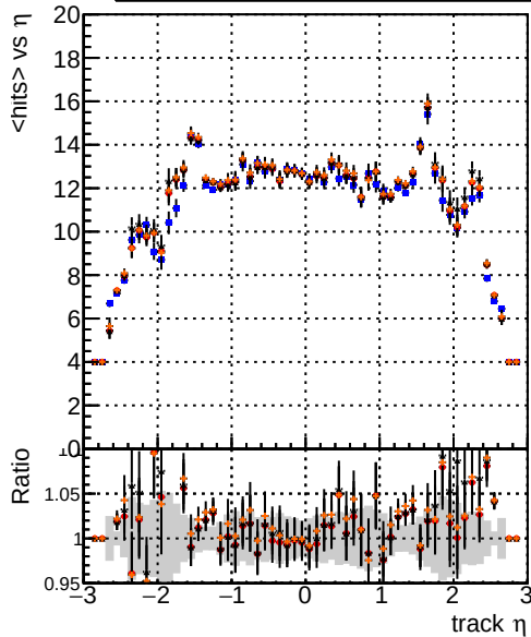
mean hit DQMstep3 TT CKF DQMstep3 TT default DQMstep3 TT ckfPixelLess DQMstep3 TT default1
