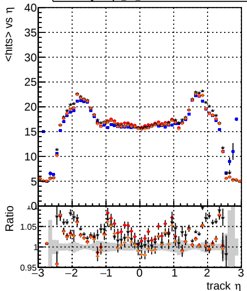
mean hits vs \eta DQMstep3 TT CKF DQMstep3 TT default DQMstep3 TT ckfPixelLess DQMstep3 TT default1
