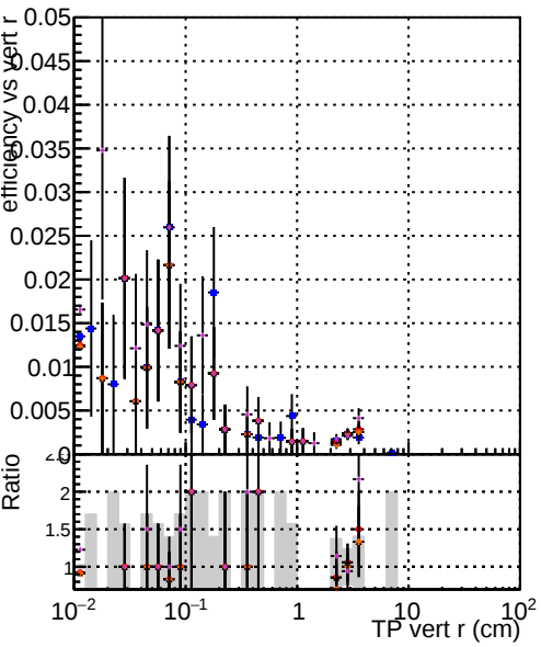
Efficiency vs TP vert r (cm) DOMstep3 CKF DOMstep3 default DOMstep3 ckrPixelLess DOMstep3 default1 DOMstep3 defaultNEWTOLDSAMPLE
