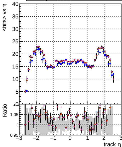
mean hits vs \eta DOMstep3 TT CKF DOMstep3 TT default DOMstep3 TT ckPixelLess DOMstep3 TT default1 DOMstep3 TT default1NEWTOLDSAMPLE
